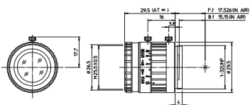
HF16HA-1B
