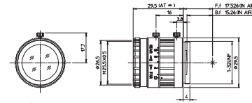
HF50HA-1B
