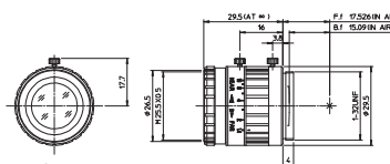
HF12.5HA-1B
